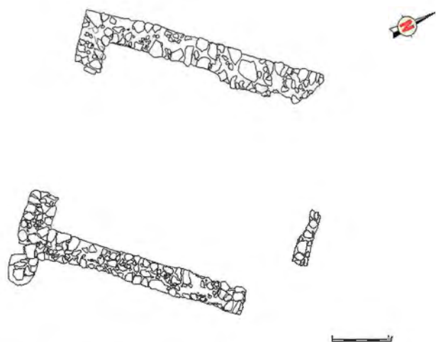
Figura 4. Planta de l'edificació de la fase I.
